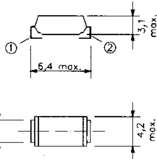
D42/SOD-6
